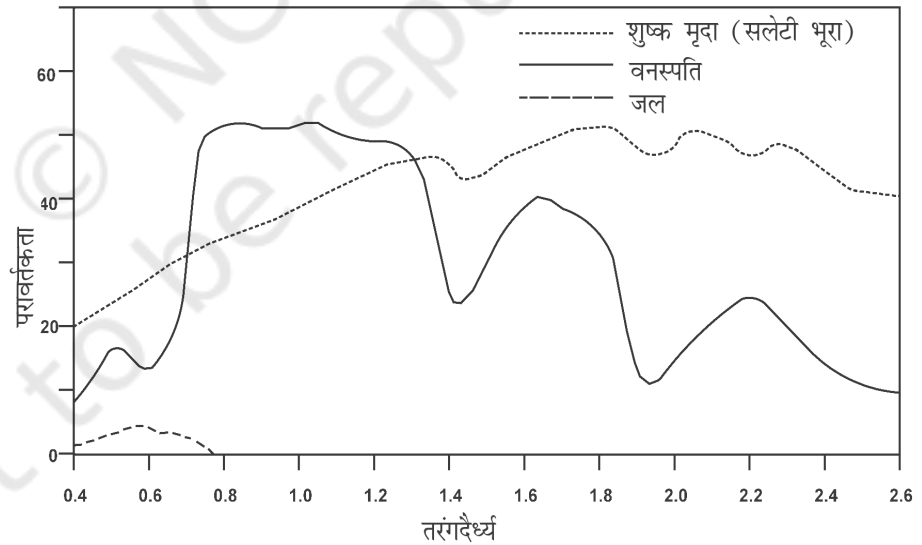
चित्र 7.5 : मृदा, वनस्पति एवं जल के स्पेक्ट्रमी चिह्नक
