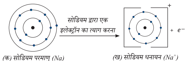
चित्र 9.11— सोडियम धनायन का निर्माण
