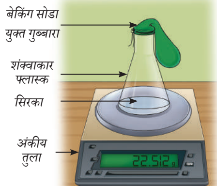
चित्र 9.3 — (क) सिरका और बेकिंग सोडा का भार
